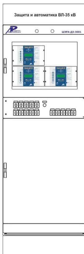
Шкаф дистанционных защит и АУВ линий 6 -35 кВ ШЭРА-ДЗ-3001 БПВА.656457.483, БПВА.650645.001 ТУ
